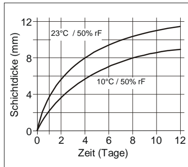
Diagramm 1: Durchhärtungsgeschwindigkeit für Sikaflex®-221
