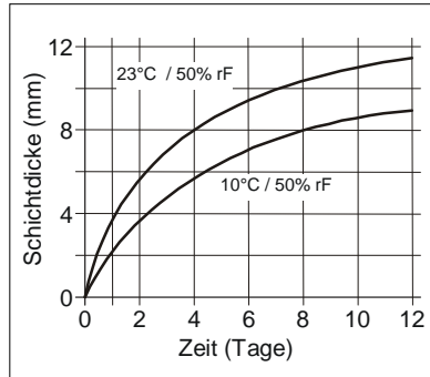
Diagramm 1: Durchhärtungsgeschwindigkeit für Sikaflex®-521 UV
